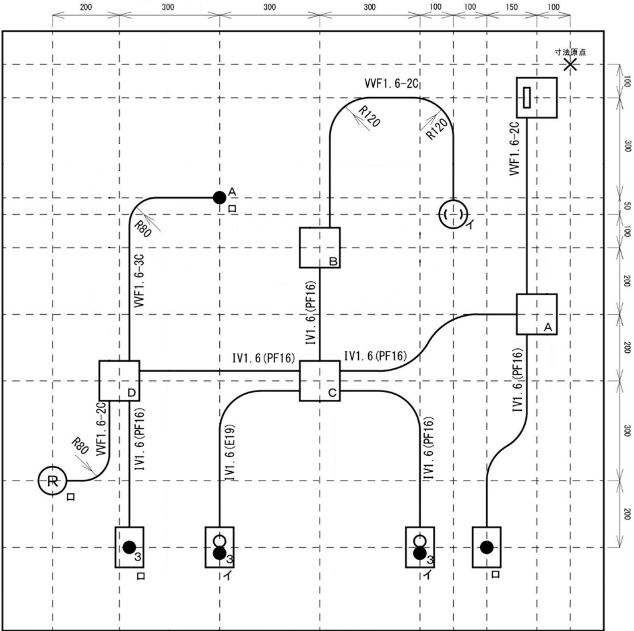
【施工図】
