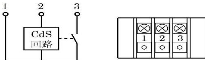
内部結線図
