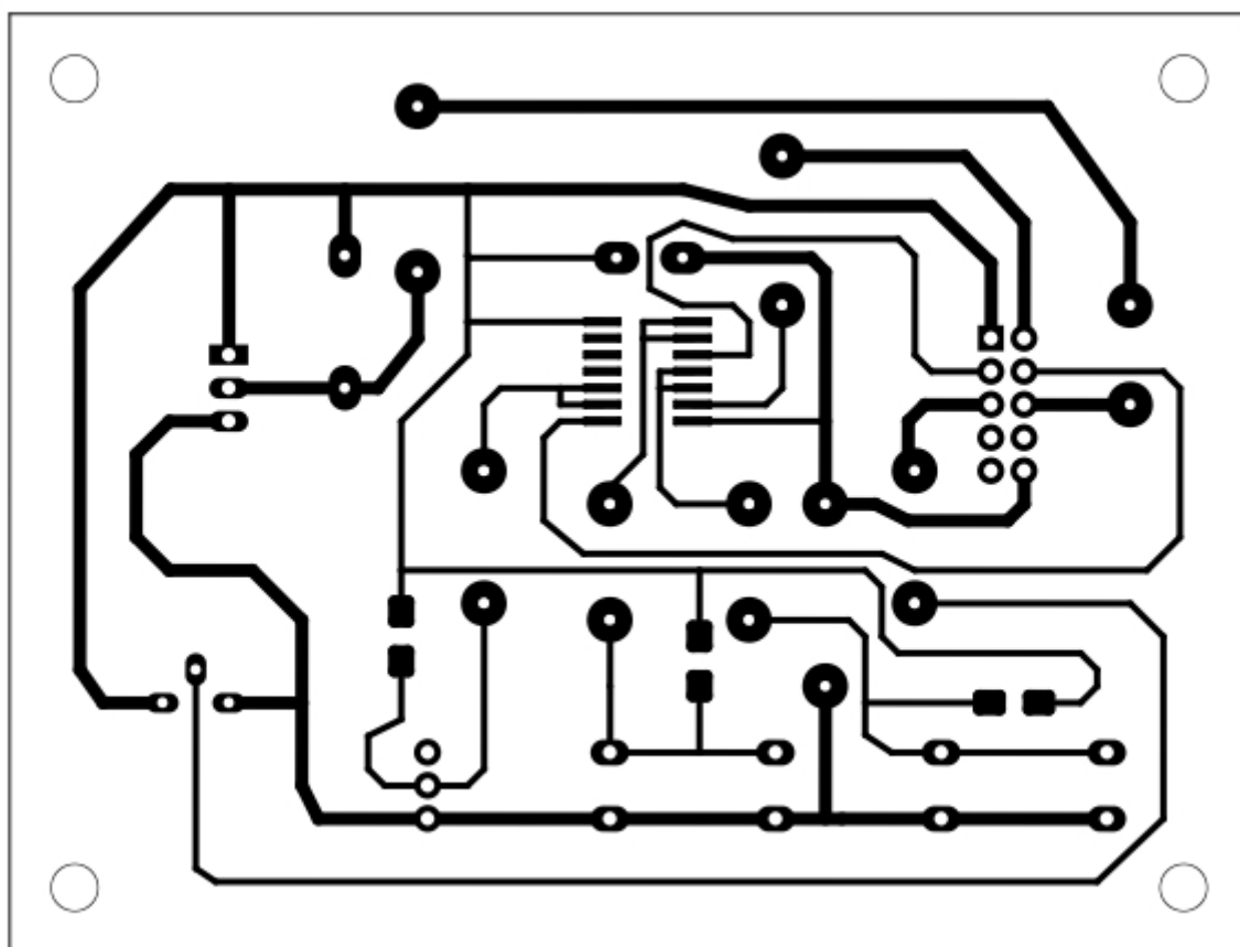
図2-b 入力回路パターン
