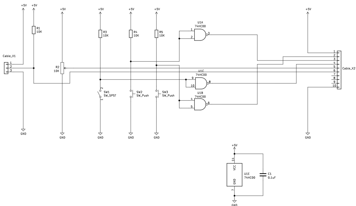
図2-a 入力回路
