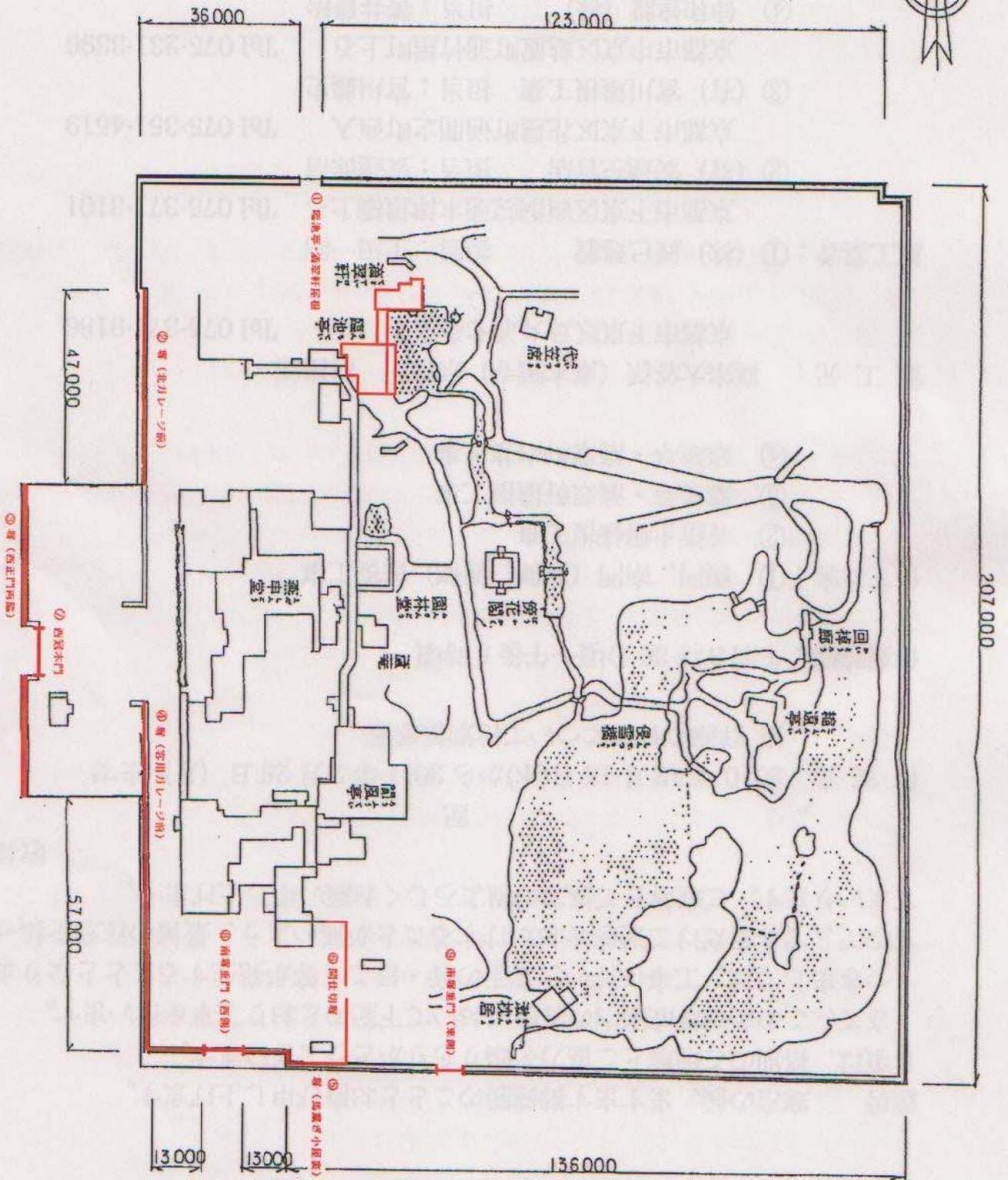
涉成園 (枳殻邸) 配置図
