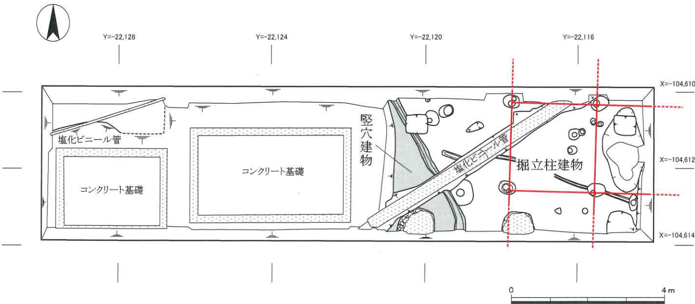
図5 遺構平面図（1：100）
